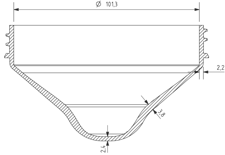
SECTION A-A
